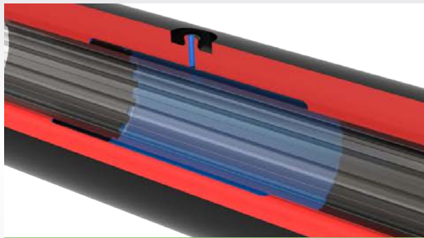
Geräumtes Schiebestück mit einem großen Fettspeicher
